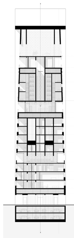
PL.5\ SECTION
