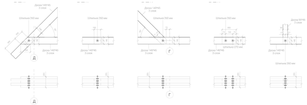
PL.3\ JOINTS [BY I.BEDNIK]
