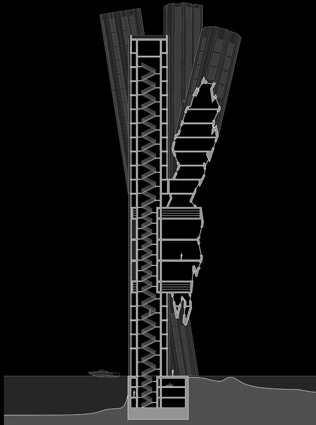
PL.4\ SECTION
